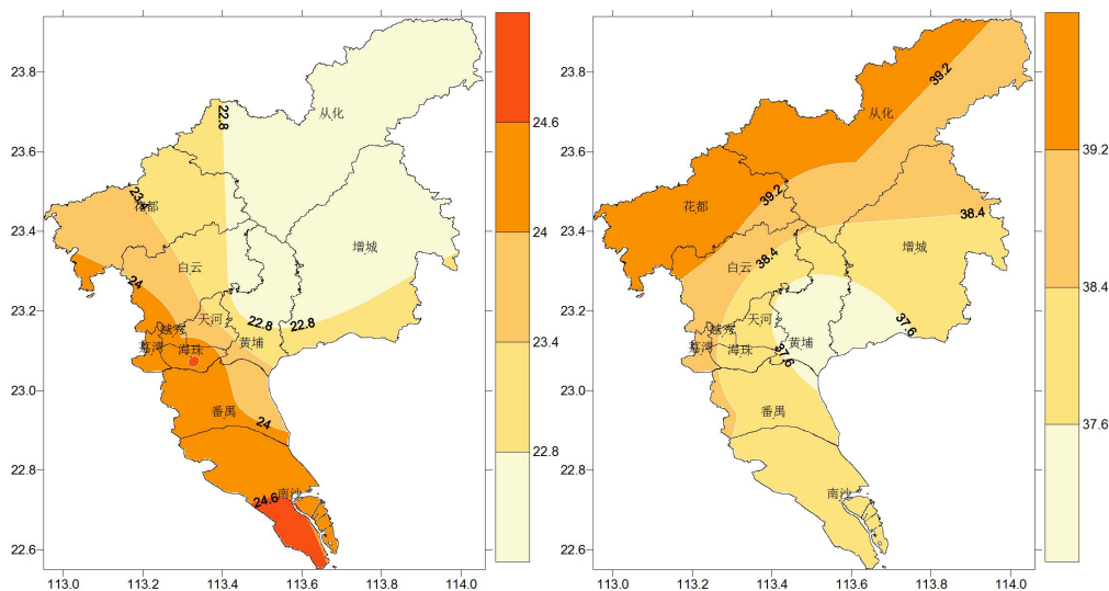
图1 2024年11月4日-11月10日广州市日平均气温（左图，单位： ^{\circ}\text{C} ）和累计日照时数（右图，单位：小时）分布图
