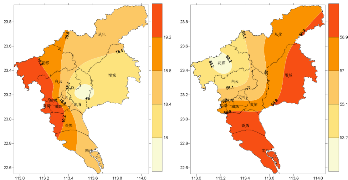
图 1 2022 年 2 月 25 日~3 月 3 日气温（左图，单位： ^{\circ}\text{C} ）和累计日照时数（右图，单位：小时）分布图
